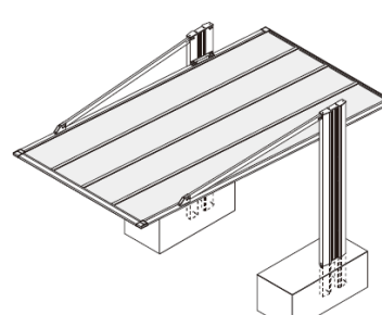
5.10) Montage Dachplatten 5.11) Montage Schutzkappen
