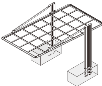
5.8) Fundamente mit Beton füllen 5.9) Fixierung Abstandhalter & Seitenprofil
