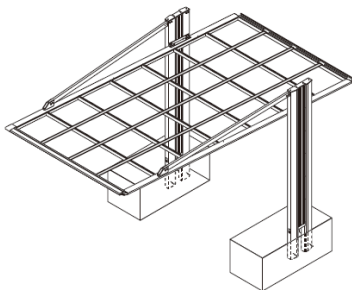
5.12) Montage Trägerschutz
